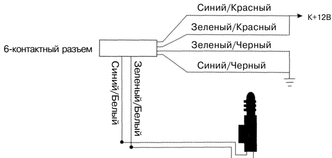
Схема 6. Установка дополнительных электроприводов
